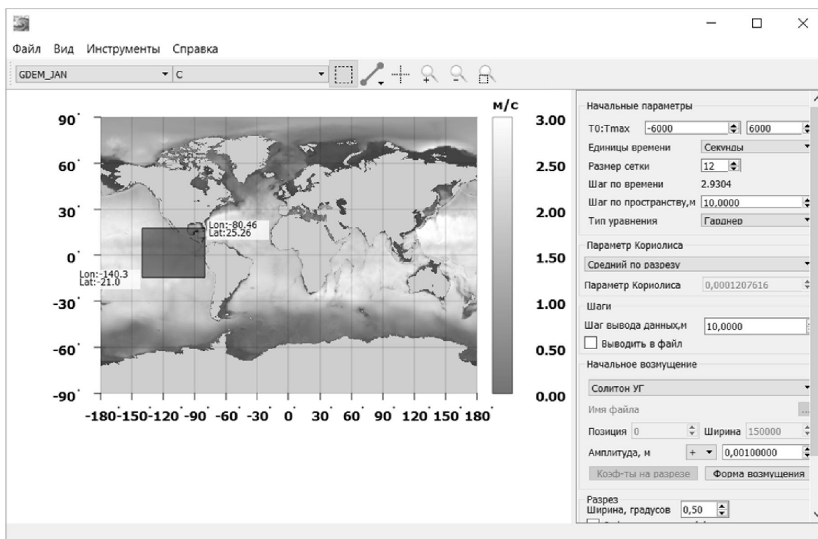
Рис. 2. Пользовательский интерфейс
