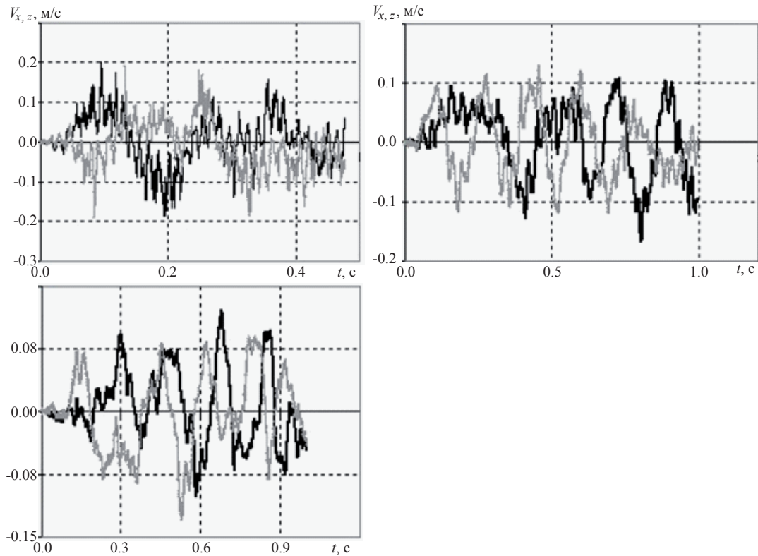
Рис. 6. Графики поперечных компонент скорости пузырьков разных диаметров: a — 3 мм; b — 5 мм; в — 10 мм (черный — V_x ; серый — V_z ).
