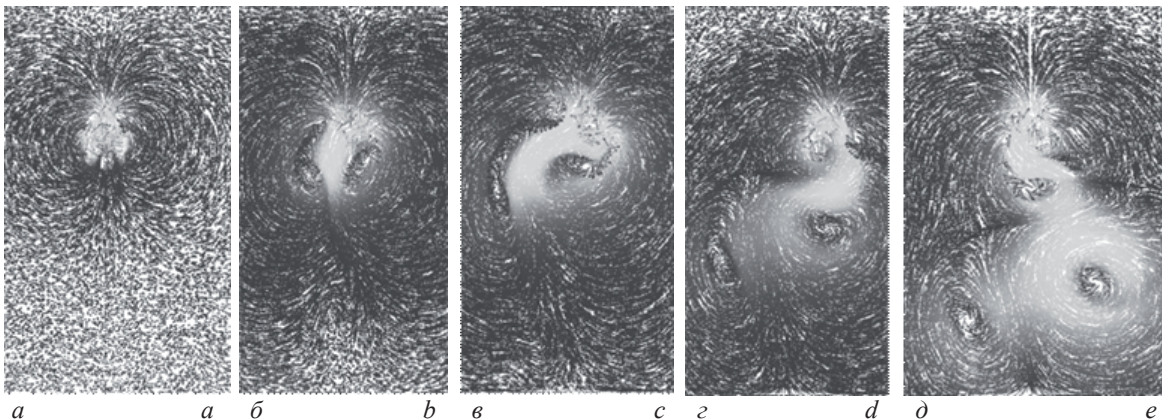
Рис. 1. Поле скорости для пузыря диаметром d = 5 мм в различные моменты времени: a — 0.05 с; b — 0.15 с; в — 0.21 с; г — 0.4 с; д — 0.47 с (масштаб кадров: ширина — 6 диаметров, высота — 10 диаметров).
