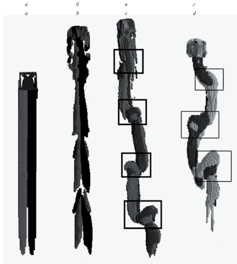
Рис. 9. Характерные вихревые следы, остающиеся за движущейся сферой: а — d = 5 мм; б — d = 7 мм; в — d = 10 мм; г — d = 20 мм.
