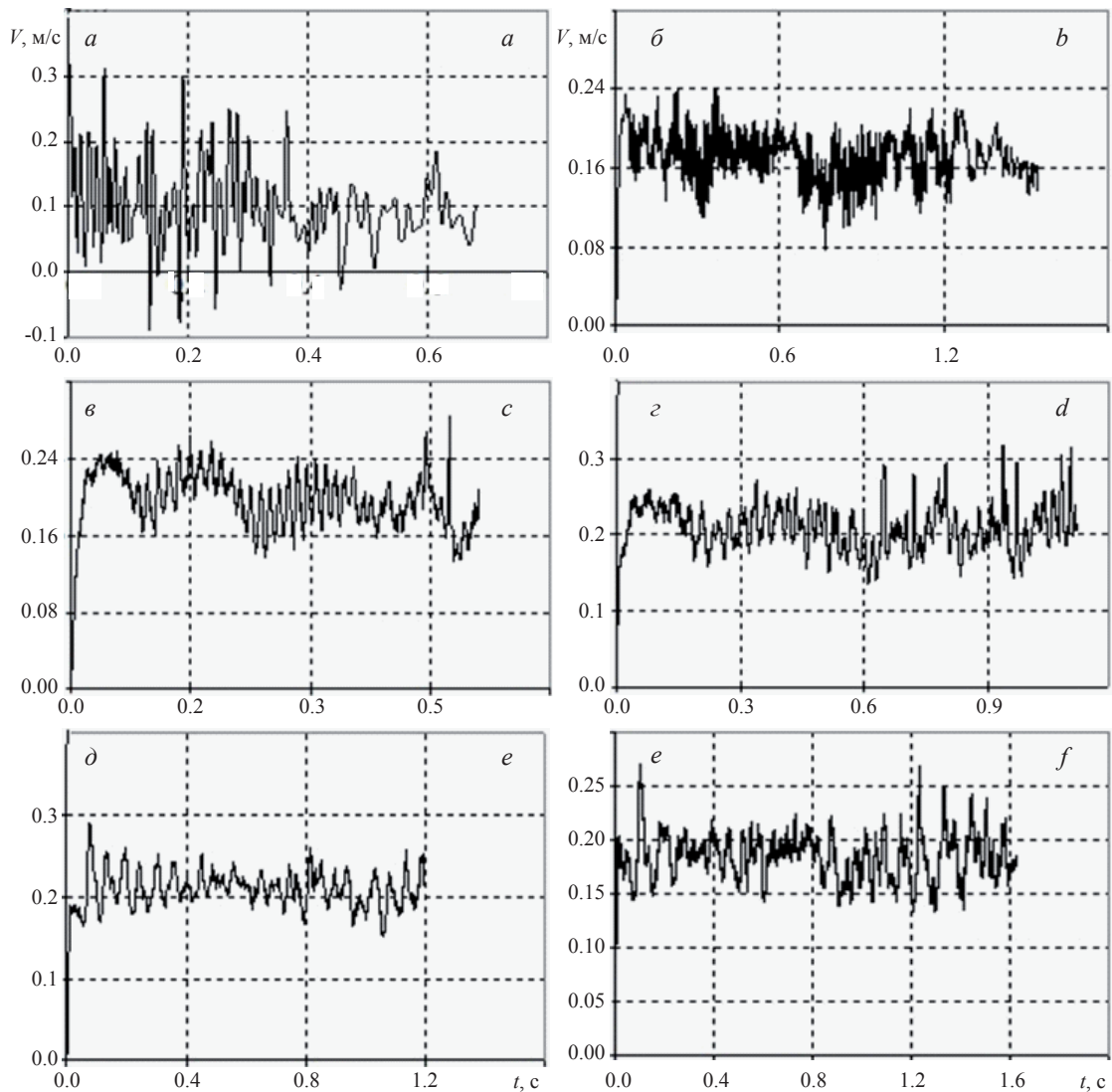
Рис. 3. Временные зависимости скорости всплывания пузыря различного диаметра d : a — 1 мм; b — 2.5 мм; c — 3 мм; d — 5 мм; e — 10 мм.
