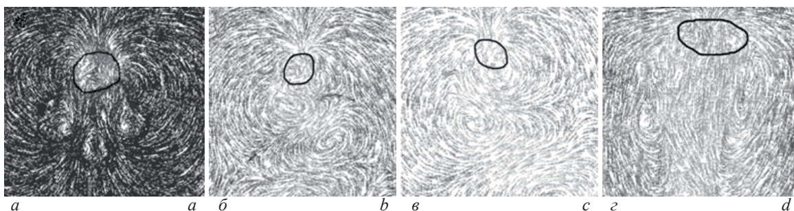
Рис. 2. Поле скорости для пузырей различного диаметра d : a — 1 мм; b — 3 мм; в — 5 мм; г — 10 мм (граница пузыря показана черной линией).
