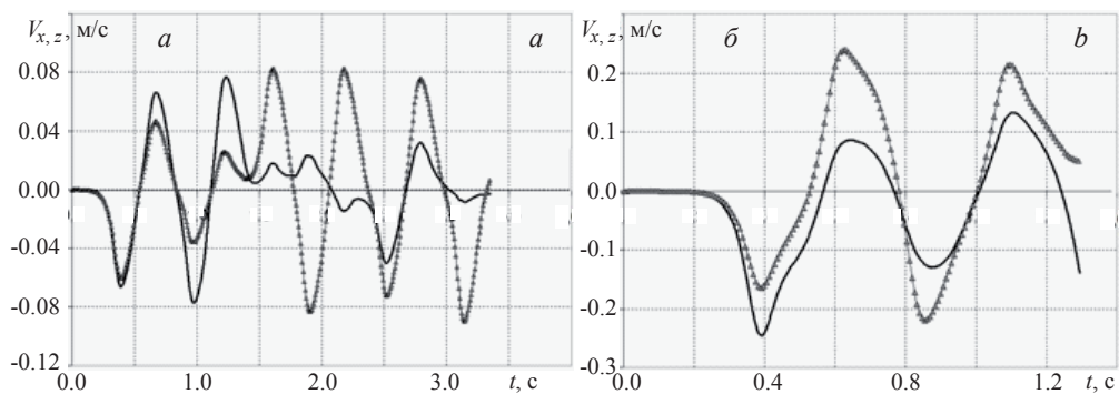
Рис. 10. Графики поперечных компонент скорости в зависимости от времени: а — d = 10 мм; б — d = 20 мм (черный — V_x ; серый — V_z ).
